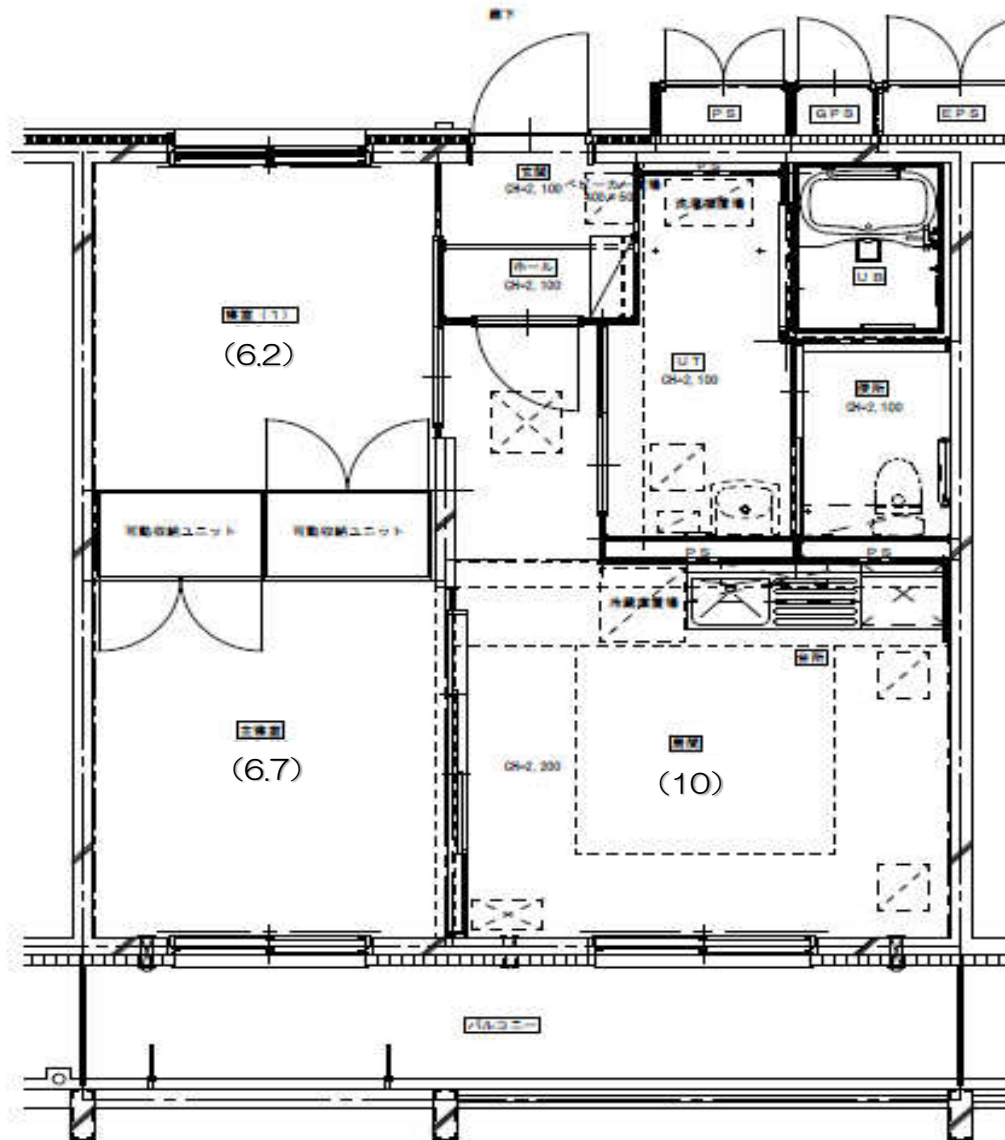
平面詳細図 (2LDK) Type 2
